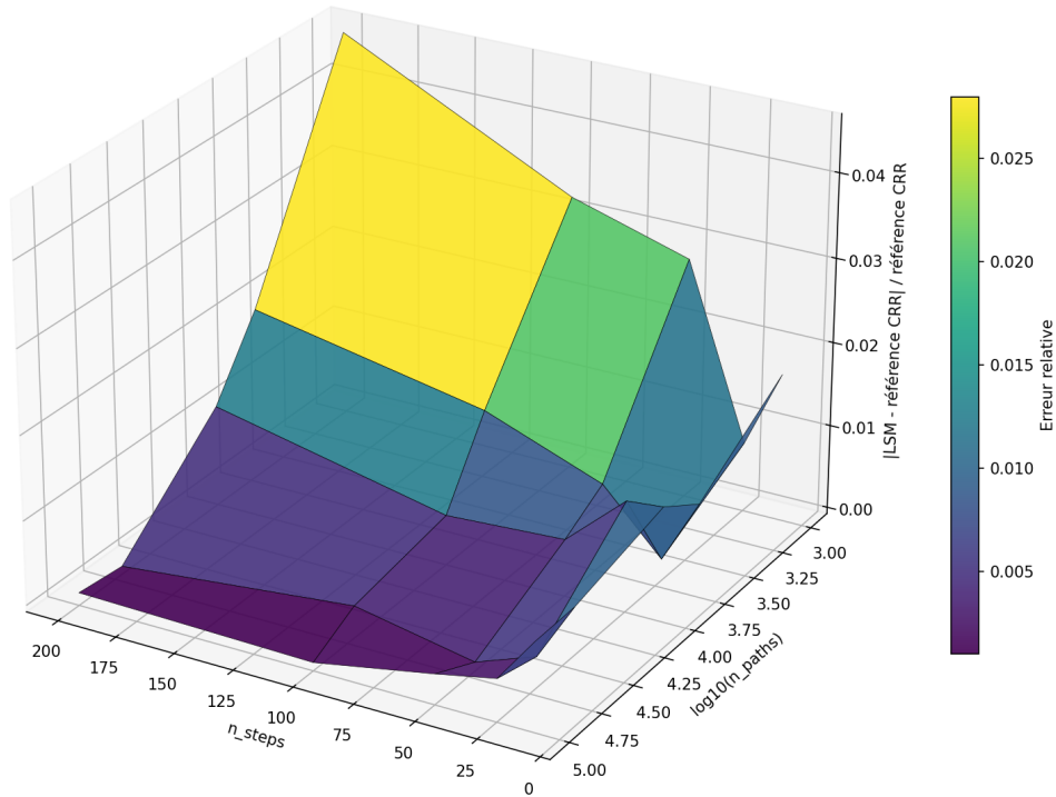
FIGURE 28 — Surface d'erreur relative en fonction de (n_{\text{steps}}, \log_{10}(n_{\text{paths}}))
