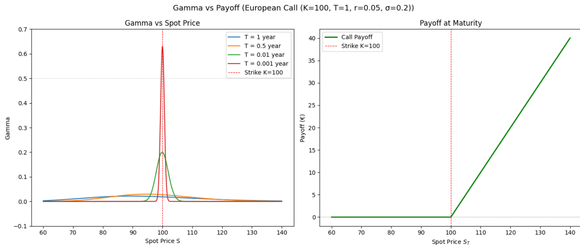
FIGURE 19 – Convergence du Gamma vers la Maturité (Call Européen)
