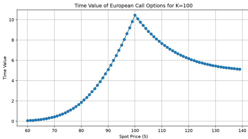
FIGURE 14 – Valeur temps d'un call européen en fonction du prix spot ( K = 100 , T = 1 an, r = 5\% , \sigma = 20\% )
