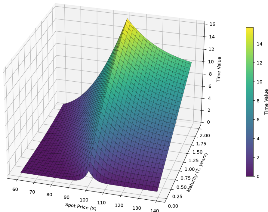
FIGURE 15 – Surface de valeur temps d'un call européen en fonction du prix spot et de la maturité ( K = 100 , r = 5\% , \sigma = 20\% )
