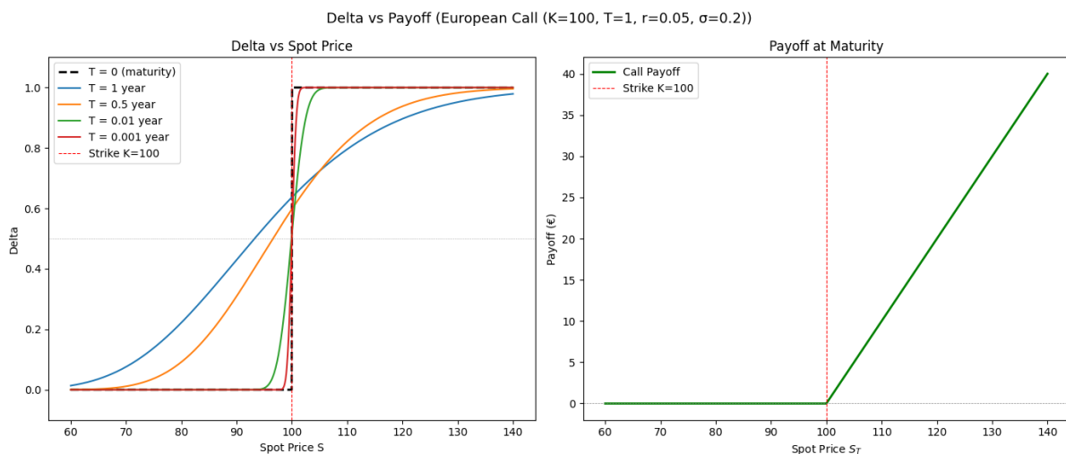
FIGURE 16 – Convergence du Delta vers la Maturité (Call Européen)
