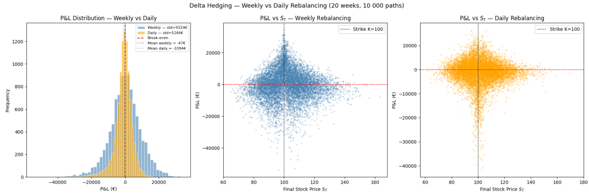
FIGURE 18 – Delta Hedging - Rééquilibrage Hebdomadaire vs Journalier sur 20 Semaines
