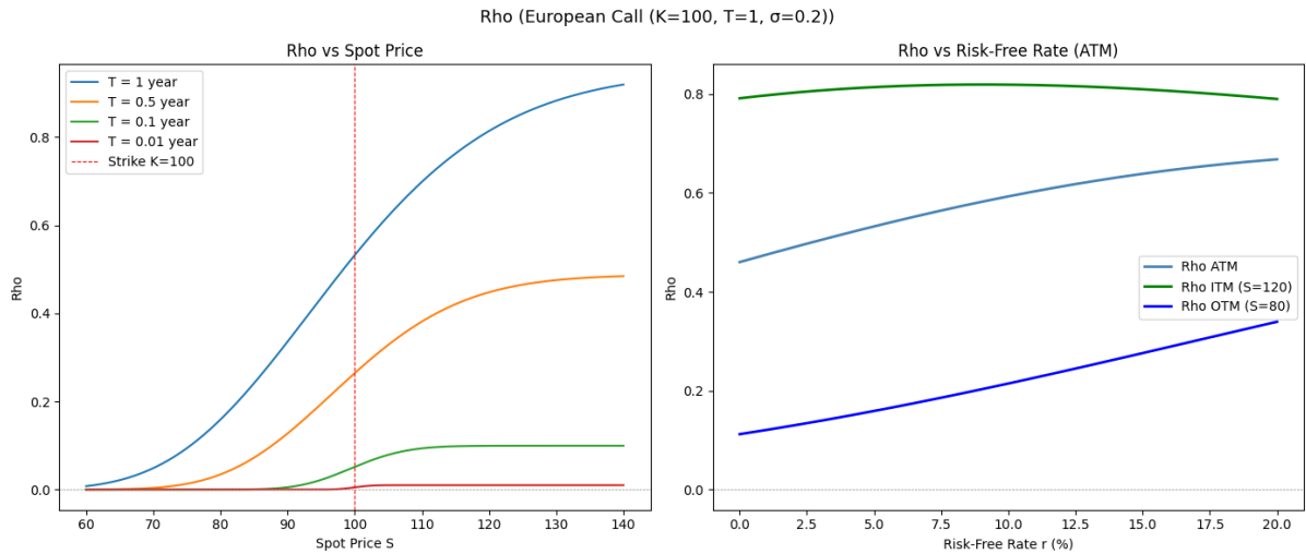
FIGURE 22 – Sensibilité du Rho aux Taux - Call Européen
