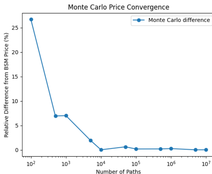
FIGURE 23 – Convergence de l'erreur résiduelle en fonction du nombre de simulations pour la méthode de Monte Carlo naïve.
